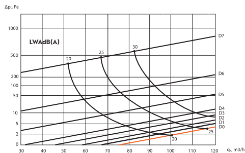
LINEO PRO 20 mm plyšys (oro tiekimas)
