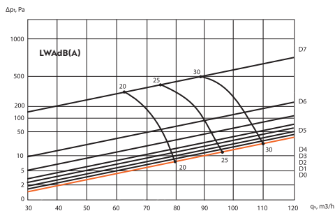
LINEO PRO 20 mm plyšys (oro ištraukimas)
